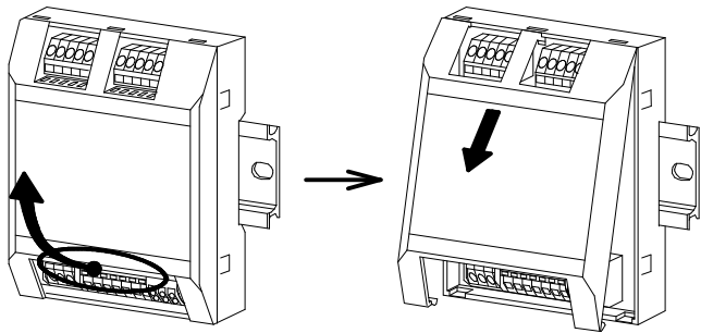
カバー下部に指を当て矢印方向に引き上げます 矢印方向にカバーを引き抜きます
