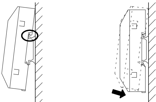
本体裏、上側の爪をDINレールに引っ掛けます パチンと音がするまでDINレールに押し込みます
