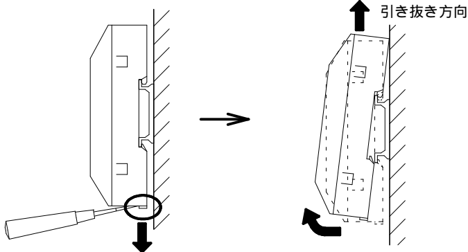
マイナスドライバを本体下部の固定具の穴に通し固定具を下方方向に動かします 本体を手前に引き上げ上部方向に引き抜きます
