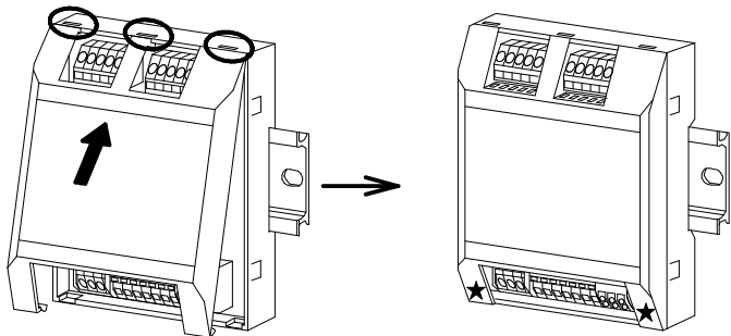
本体上部の溝(3箇所)にカバー上部の爪を差し込みます 部を押し込み下部の爪をはめ込みます
