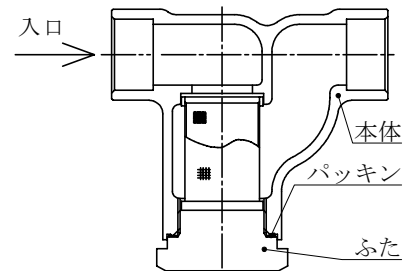
ろう付形
